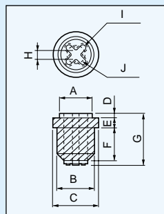
寸法図
