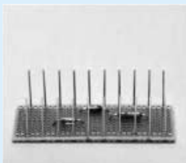
プリント基板に部品とピンを取付けて半田付する。
