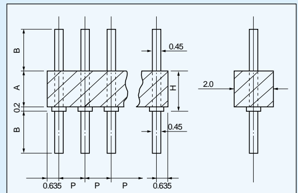
寸法図
