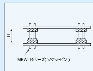
H寸法はMXW-1シリーズとMEW-1シリーズ(74ページ参照)を組合せた時のプリント板同志の間隔です。
