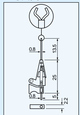
寸法図
